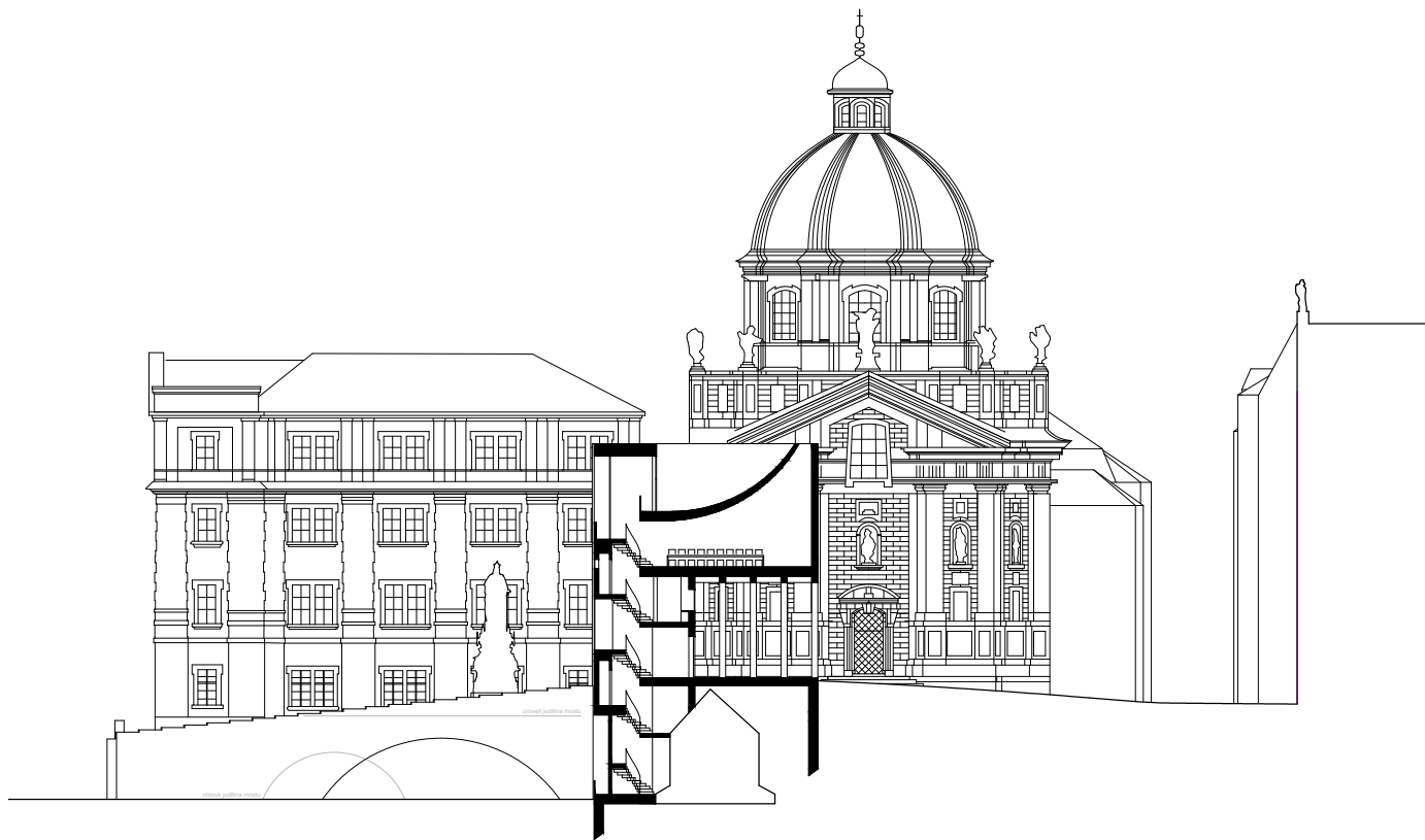
SNITT A-A
