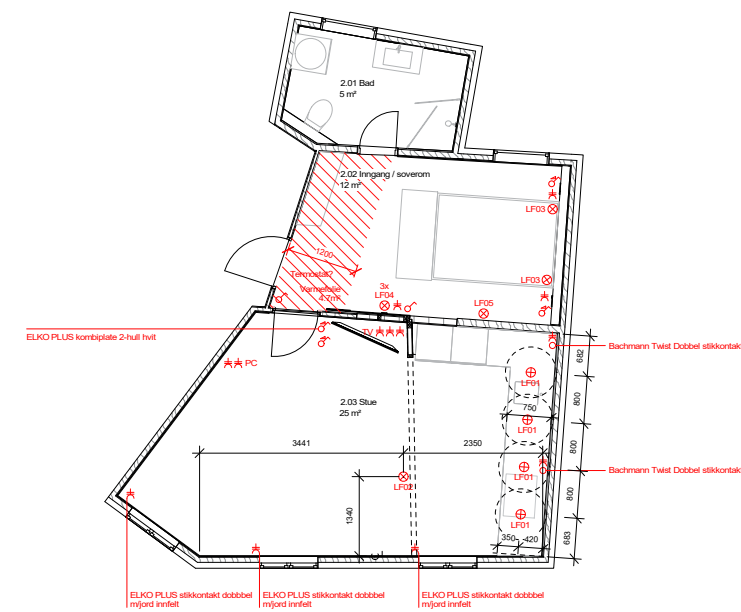
ELEKTROPLAN
